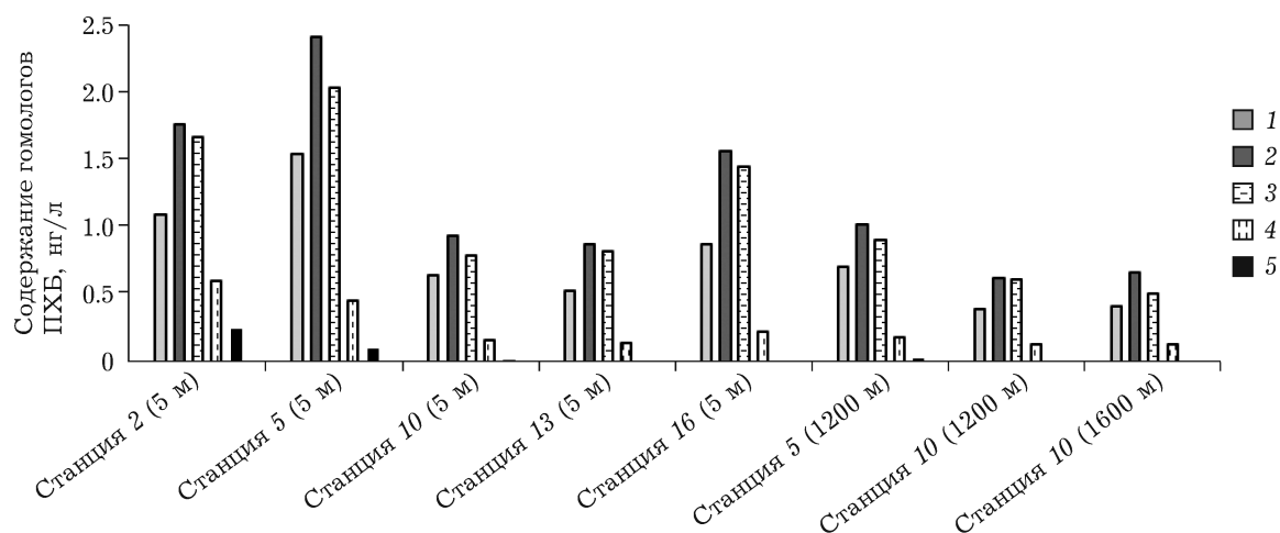
Рис. 2. Соотношение групп гомологов ПХБ в верхних и глубинных водных горизонтах: три- (1); тетра- (2); пента- (3); гекса- (4); гептахлорированные (5) бифенилы.
